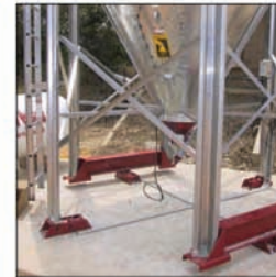
Silos con células de carga
